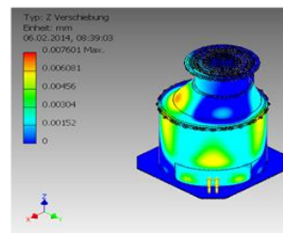
Comprobación FEM
